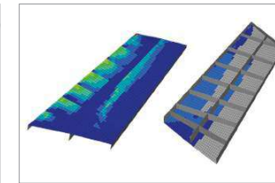
평면요소 상관과 하단의 컨투어를 동시에 확인
