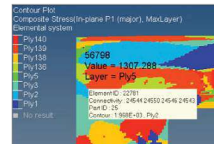
복합재료에 특화된 후처리 기능
