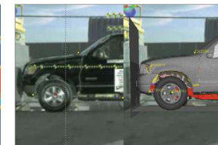
오차를 최소화한 CAF - 실제 시험 비교
