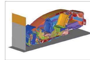
단면도 확인을 통한 간섭 확인
